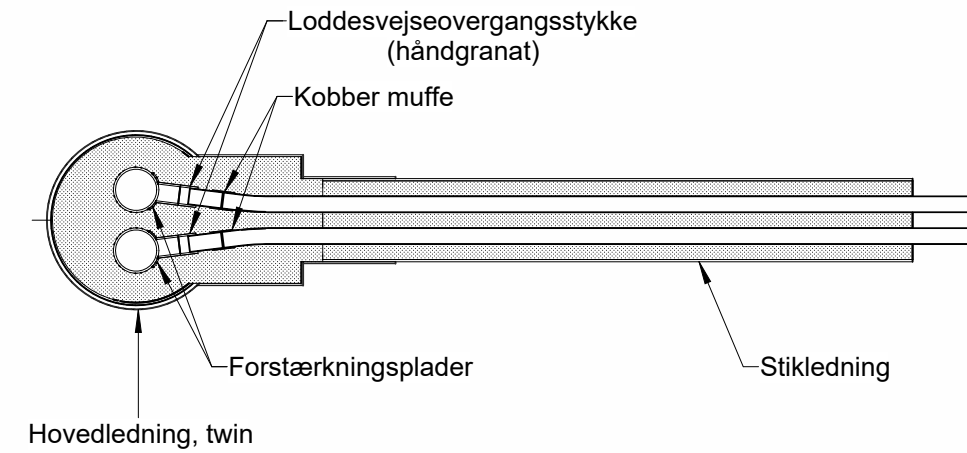
SNIT A-A
