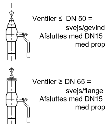
Detalje 1
