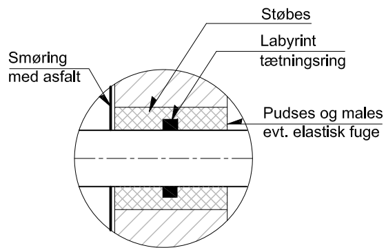
Detalje 1
