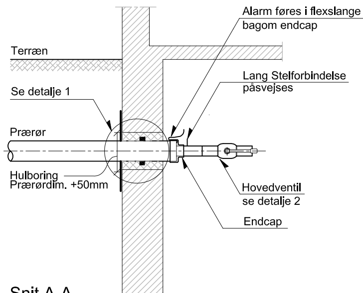
Snit A-A
